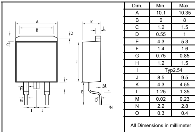
T0-263
